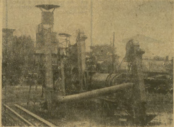
Oto zespół do suszenia i otaczania kruszywa, który w przeciągu godziny przygotowuje 25 ton masy dla budowy nowoczesnej nawierzchni drogowej.
