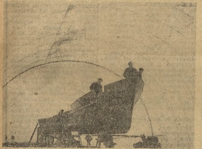
We wnętrzu namiotu, który zastępuje halę produkcyjną odbywa się powlekanie lakierem kadłuba statku.
