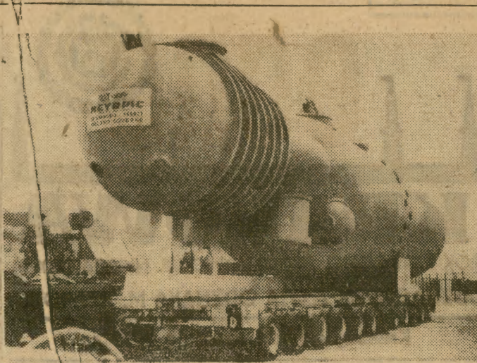
Budowa francuskiej kabiny podwodnej „Argyronete” zostanie ukończona w 1973 r. Urządzenie to wykorzystane będzie przy poszukiwaniach ropy naftowej oraz badaniach naukowych, a także w akcjach ratowniczych. N.Z: dwa stalowe kadłuby „Argyronete”. CAF — AFP
