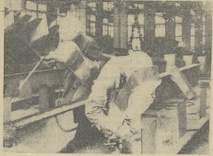
Załoga Stoczni im. Komuny Paryskiej w Gdyni przystąpiła do wyłączonej pracy. Na zdjęciu: na Wydziale K-3 Montażu Kadłubów, spawacze przy montażu sekcji pokładu.
