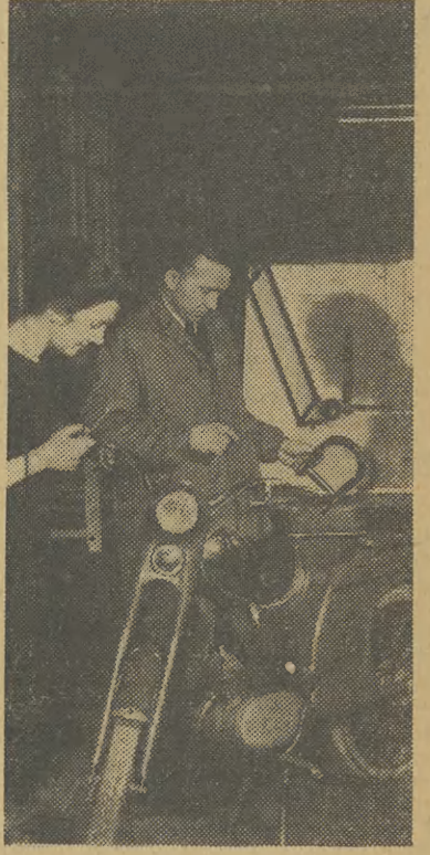
Zakłady Metalowe Wrocław-Zakrzów rozpoczynają seryjną produkcję motorowerów typ MR-1. Na zdjęciu: pracownicy biura konstrukcyjnego zakładów pod kierunkiem inż. Zbigniewa Domicza przeprowadzają badania motoroweru.
