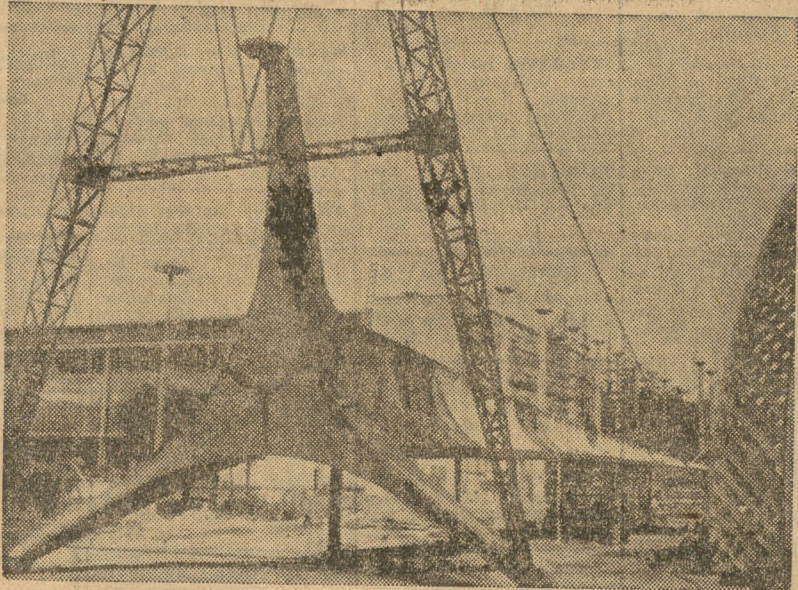
Fot. Ag. „Od A do Z” — E. Węglowski Igllica — symbol Wystawy — przed ustawieniem. Wysokość konstrukcji 106 m; projekt: dr inż. St. Hempel
