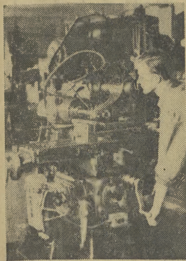
Frezer Włodzimierz Sokolowski podczas obróbki części precyzyjnej na frezarce.
