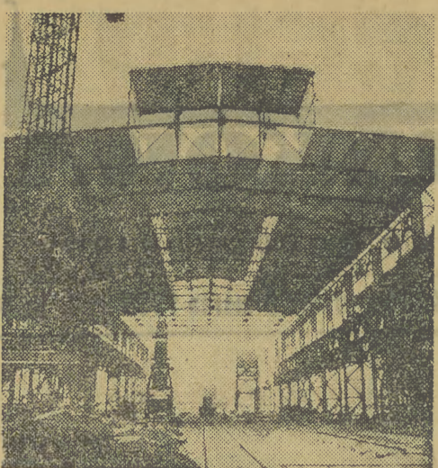
Już w polewie 1957 r. rozpocznie produkcję walcownic blach na zimno w Kombinacie Huty im. Leona Wielka hala walcowni, której budowę właśnie teraz rozpocznie, będzie posiadać ok. 1500 agregatów. Jej powierzchnia przekroczy o 40 proc. największą dotychczas halę Kombinatu-walcowni blach na gorąco. Przy budowie tego obiektu stosuje się wielkopłytowe elementy prefabrykowane.
