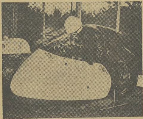
Nowy typ motocykla sportowego „S-254” wystawiony na Wszzechwłazkowej Wystawie Przemysłowej 1957 r. Posiada on dwucylindrowy czterotaktowy silnik o mocy 22 KM. Szybkość — do 150 km/godz. CAF
