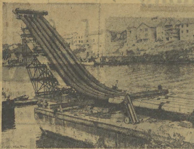
Olbrzymie rury gazowe zostaną zatopione w Sekwanie na wysokości Saint-Denis. Iśc nimi będzie gaz do Paryża.
